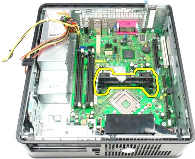
14. 卸下将系统板固定到计算机机箱的螺钉。
