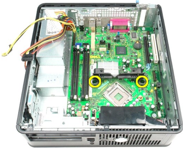
13. 卸下散热器固定模块。
